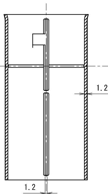
A-A 断面図
